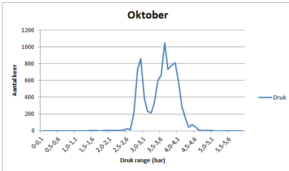
Afbeelding D.8 – aantal keer dat een druk range voorkomt in oktober bij plek I
