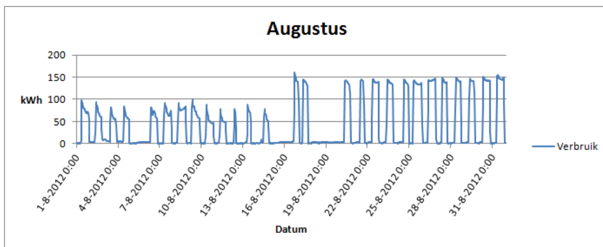
Afbeelding F.1 – Elektriciteitsverbruik GWW in augustus
