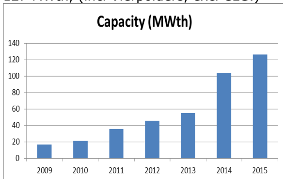
Figuur 2: totale capaciteit van de Nederlandse geothermie in MWth.
